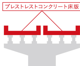
プレストレストコンクリート床版
